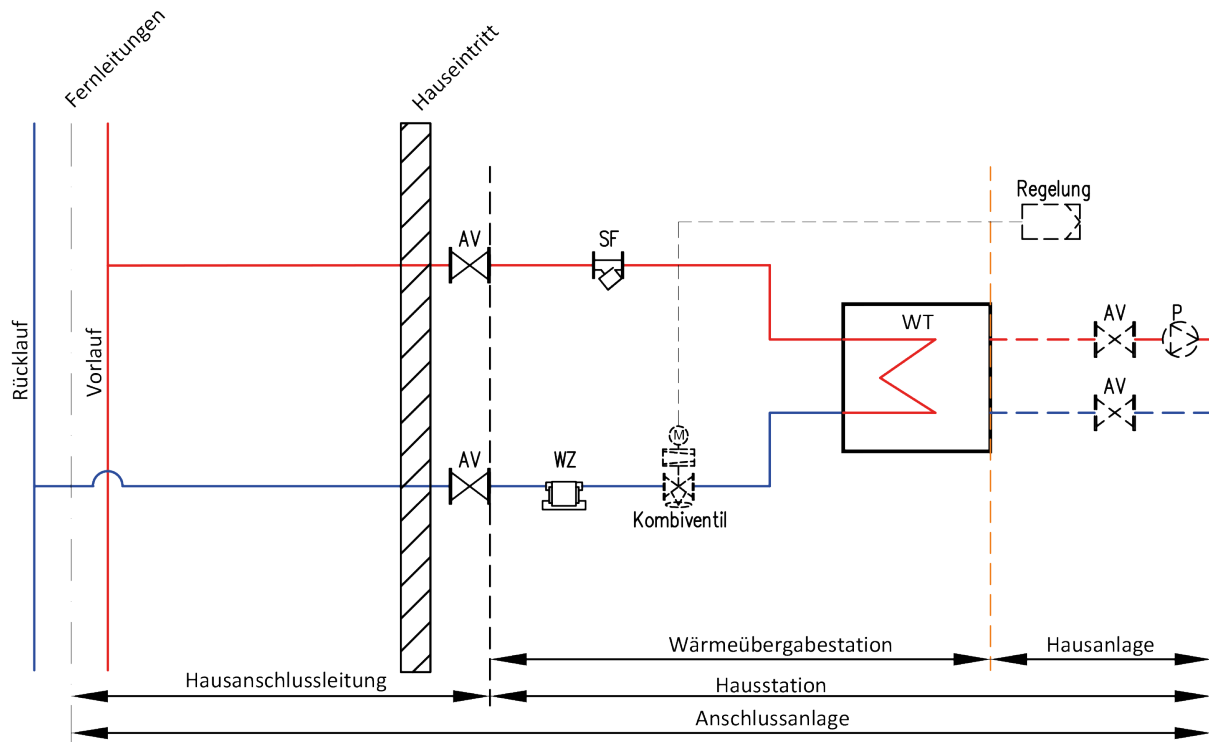
Abbildung 1: Wärmeübertragung indirekt
